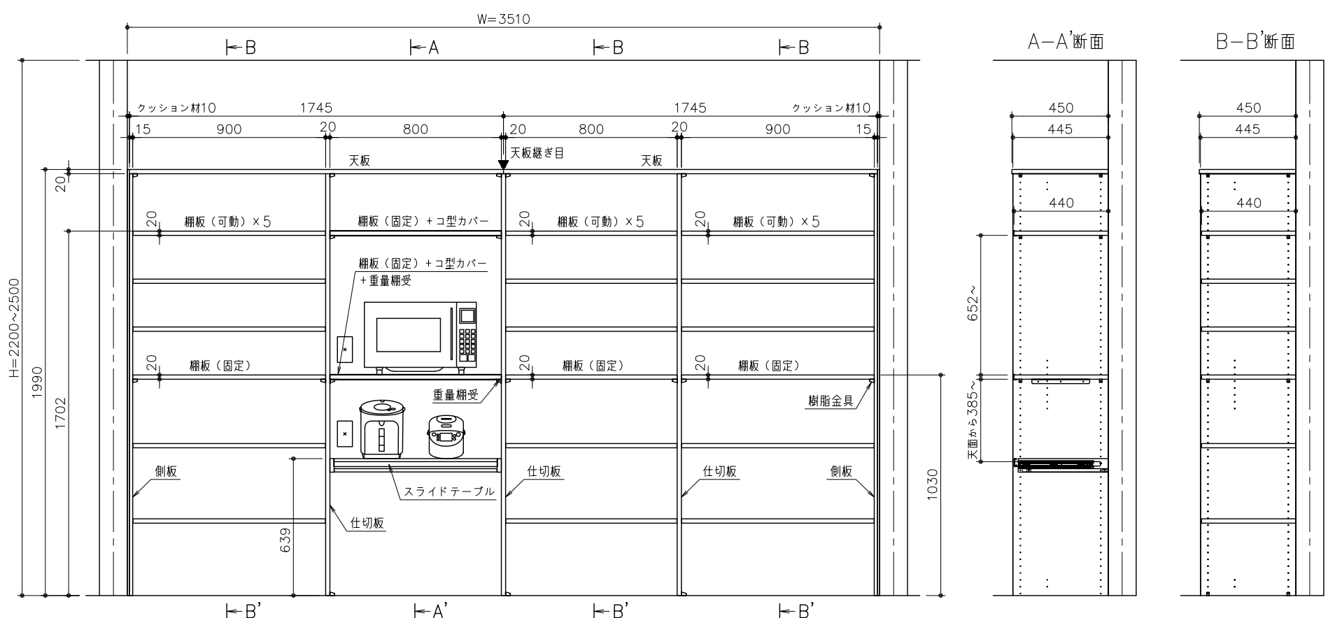
[正面図]
