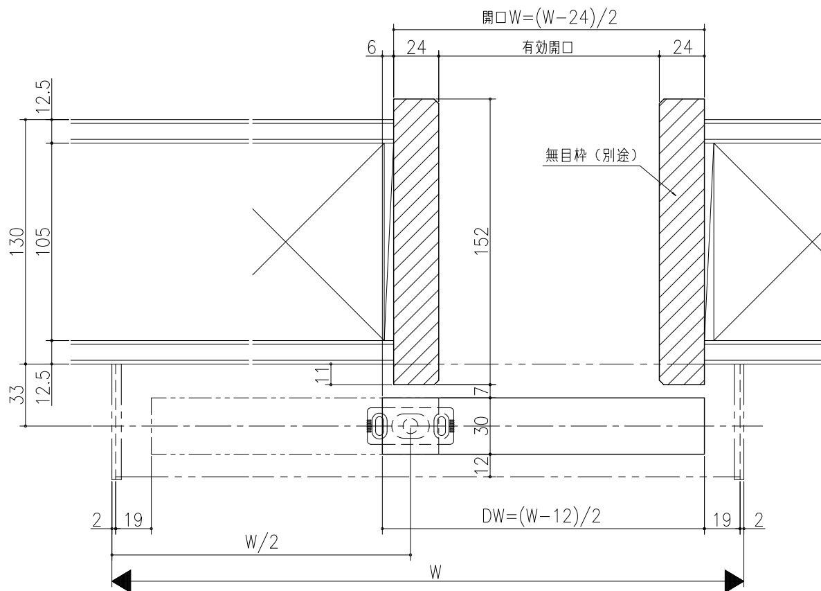
D TOS多機能商品シリーズ 室内引戸<アウトセット仕様> 片引き戸 無目枠納め(ノンケーシング枠) たて横断面 d t 28 c 0 0 1
