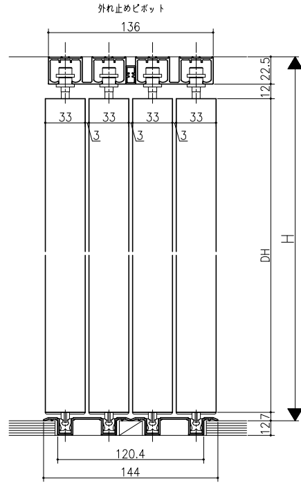
埋め込みアルミ敷居 (調整)
