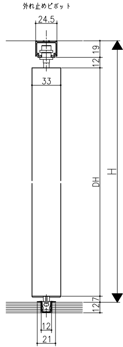
外れ止めピボット 埋め込みアルミ敷居 (調整)
